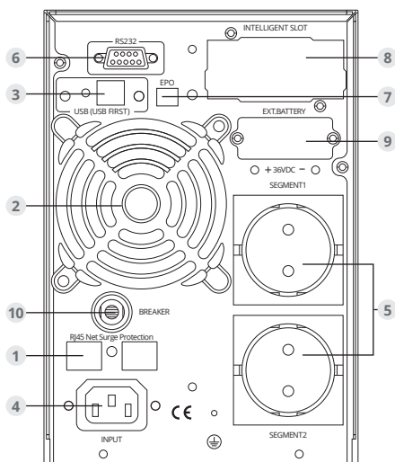
Рис. 2: Вид сзади: ИБП ИМПУЛЬС СТАЙЕР11-1 (1 кВА)
